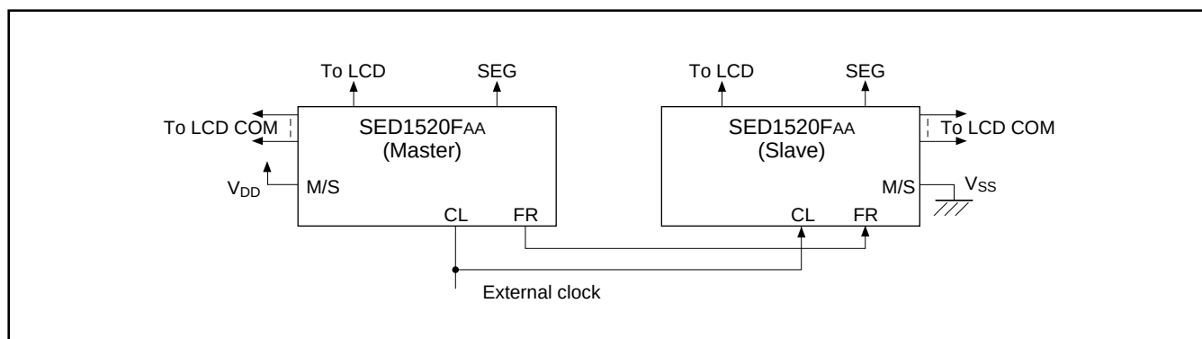
Figure 7.2. SED1520FAA – SED1520FAA
